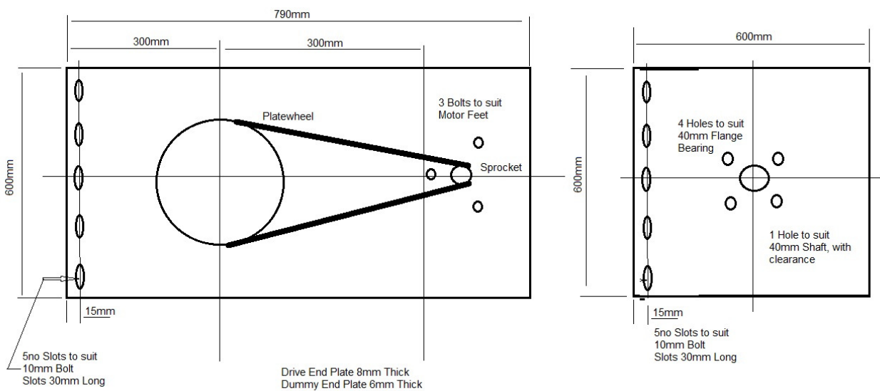
800kg Motor Endplate NF8006
