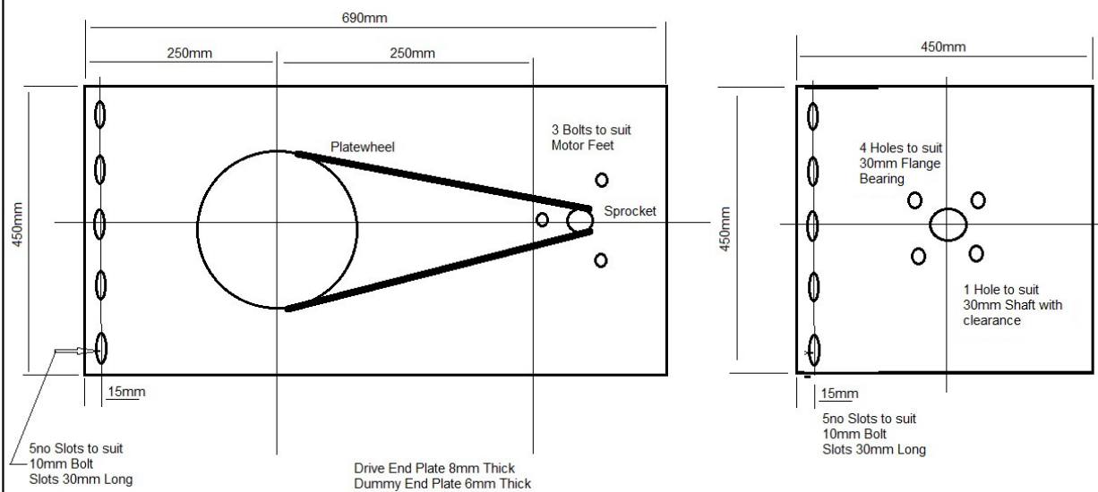
500kg Motor Endplate NF5004
