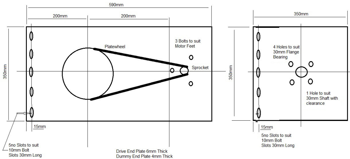
500kg Motor Endplate NF5003
