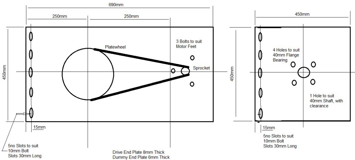
800kg Motor Endplate NF8004
